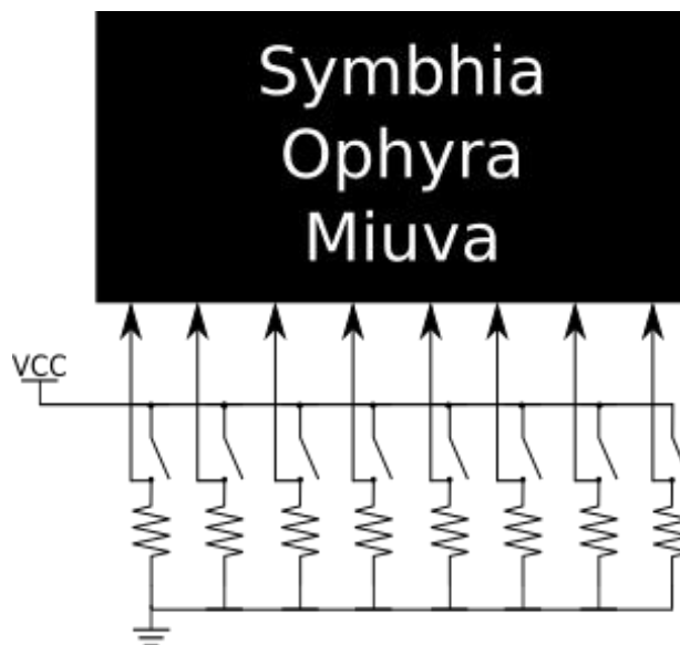
Figura1. Esquemático Simplificado
